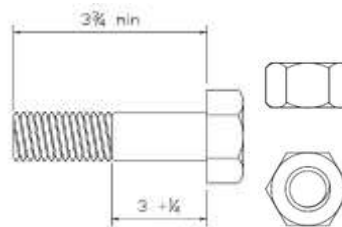
A) TAB-150-NC
