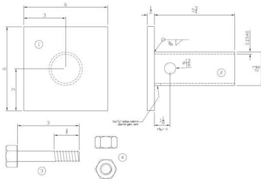
A) TAB-150-NC
