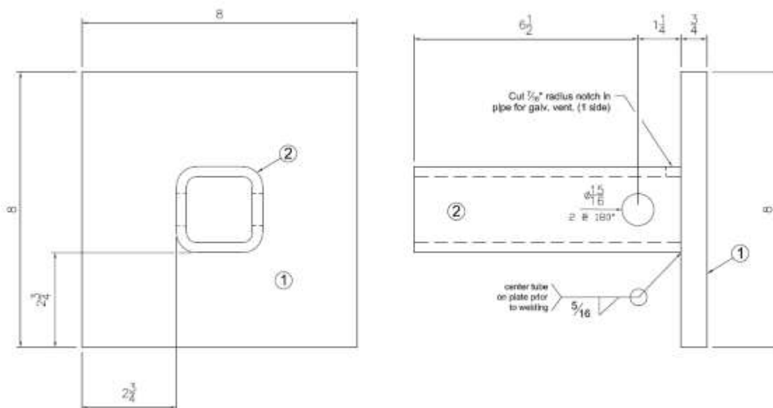
B) TAB-175-NC
